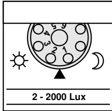
Dämmerungseinstellung (Ansprechschwelle) ⑤
