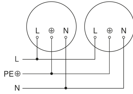
aansluitschema
