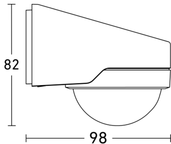
Maßzeichnung 2
