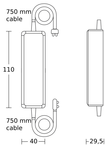
Dessin dimensionnel 2
