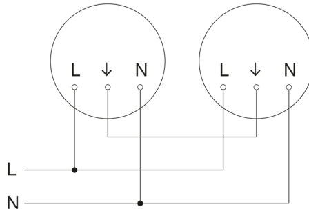
Schaltplan Master-Master Vernetzung
