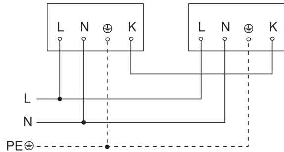
Schaltplan Master-Master Vernetzung
