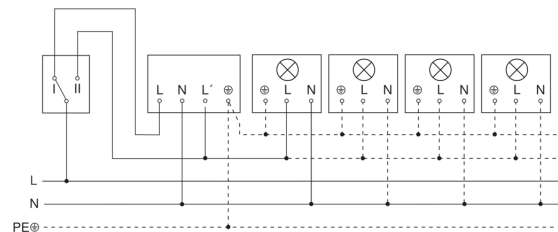
Schaltplan Anschluss über einen Wechselschalter für Dauerlicht- und Automatik-Betrieb
