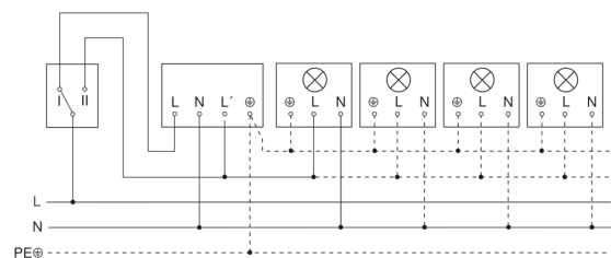
Schaltplan Anschluss 4-fach Tasterkoppler an DALI2 APC
