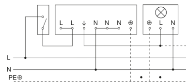
Schaltplan Master-Slave Vernetzung
