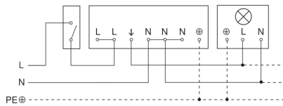
Schaltplan Master
