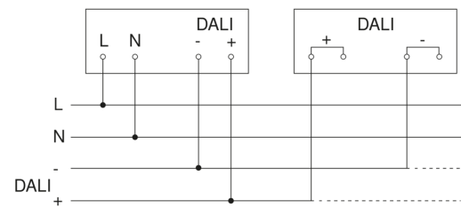
Schaltplan Vernetzung DALI-2 APC mit DALI-2 IPD
