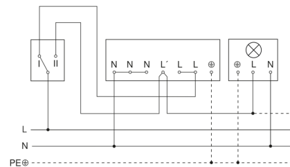
Schaltplan Anschluss 4-fach Tasterkoppler an DALI2 APC
