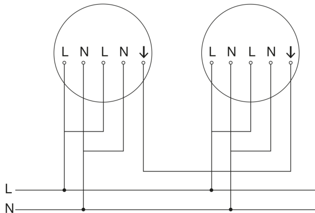
Schaltplan Master-Master Vernetzung
