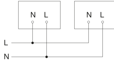
Schaltplan Master-Master Vernetzung
