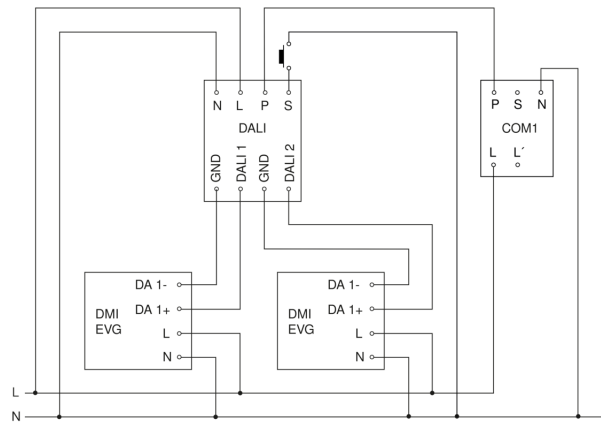
Schaltplan Master-Master Vernetzung
