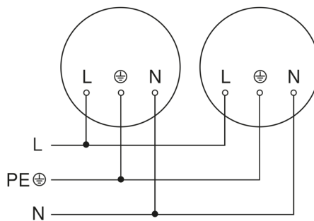
Schaltplan Master-Slave Vernetzung
