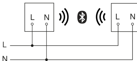
Schaltplan Master-Master Vernetzung
