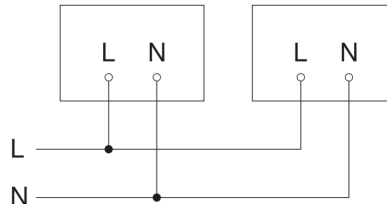
Schaltplan Master-Master Vernetzung
