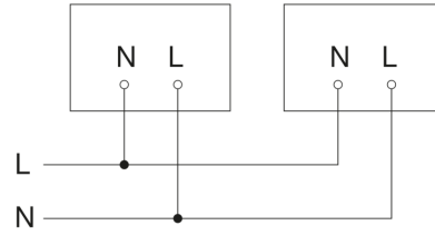
Schaltplan Master-Master Vernetzung
