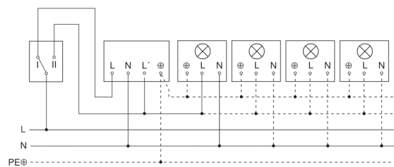
Schakelschema Aansluiting via een wisselschakelaar voor continu en automatisch bedrijf
