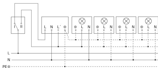
Aansluiting van 4-voudige drukknopkoppeling op DALI2 APC
