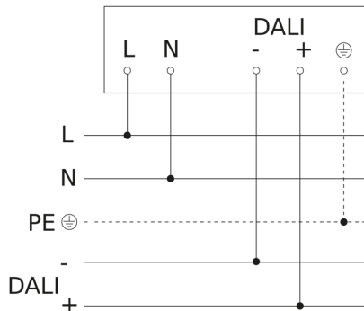
aansluitschema Master
