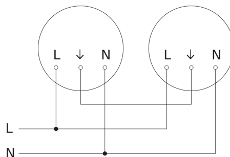
Schema elettrico Master-Master collegamento in rete
