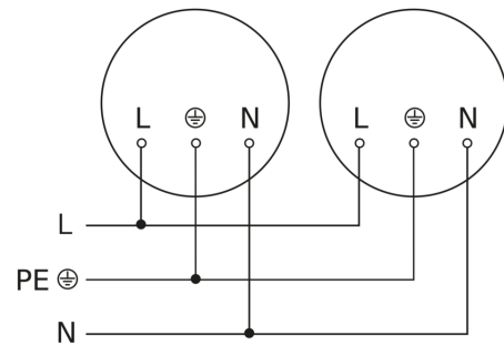
aansluitschema
