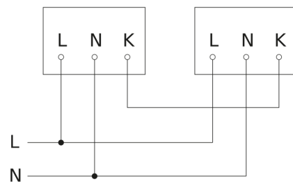
aansluitschema master/master
