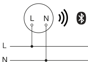
aansluitschema slave/draadloze masterkoppeling
