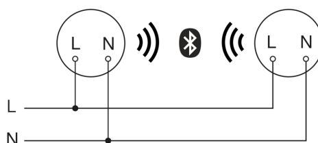
aansluitschema master/master
