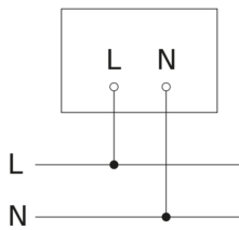
aansluitschema Master/slave koppelin
