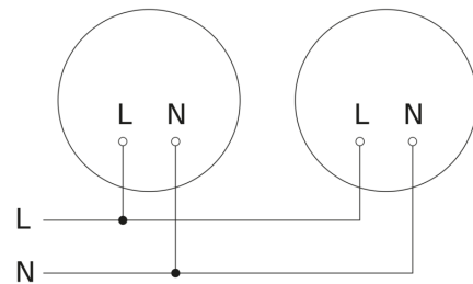
Schéma du circuit d'interconnexion maître/maître
