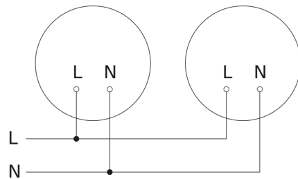
aansluitschema master/master Bluetooth
